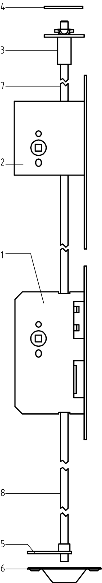
Standflügel
